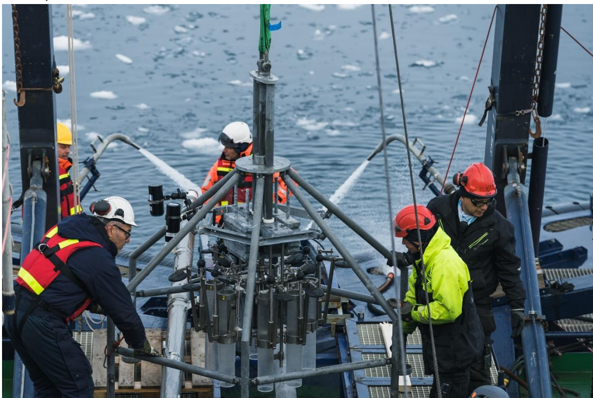
Arbete på akterdäck, sjösättning Multicorer
